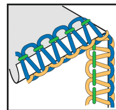
3-х ниточный узкий подрубочный шов - кайма
