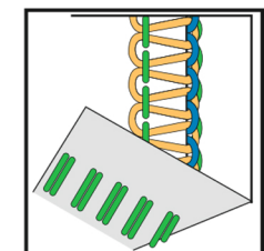
3-х ниточный узкий шов Flatlock
