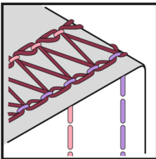
3-х ниточный широкий плоский шов
