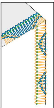
3-х ниточный обратный волновой шов
