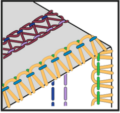
6-ти ниточный шов 3-х ниточный узкий плоский шов + 3-х ниточный ролевой шов
