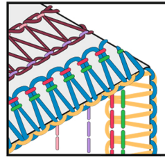
7-ми ниточный шов 3-х ниточный широкий плоский шов + 4-х ниточный оверлок
