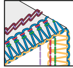
6-ти ниточный шов 2-х ниточный цепной шов + 4-х ниточный оверлок
