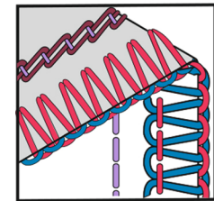
4-х ниточный шов 2-х ниточный цепной шов + 2-х ниточный широкий оверлок
