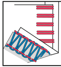
2-х ниточный декоративный шов лесенкой
