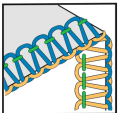
3-х ниточный узкий оверлочный шов
