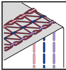
4-х ниточный плоский шов
