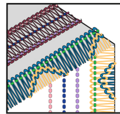
7-ми ниточный шов 4-х ниточный плоский шов + 3-х ниточный обратный волновой шов
