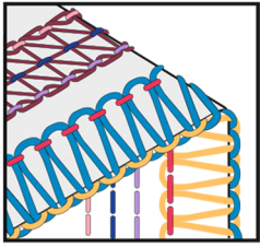
7-ми ниточный шов 4-х ниточный плоский шов + 3-х ниточный широкий оверлок
