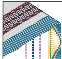
7-ми ниточный шов 4-х ниточный плоский шов + 3-х ниточный волновой шов
