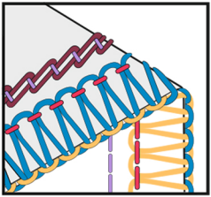
5-ти ниточный шов 2-х ниточный цепной шов + 3-х ниточный широкий оверлок
