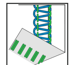
2-х ниточный узкий шов Flatlock
