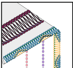
6-ти ниточный шов 3-х ниточный широкий плоский шов + 3-х ниточный ролевой волновой шов
